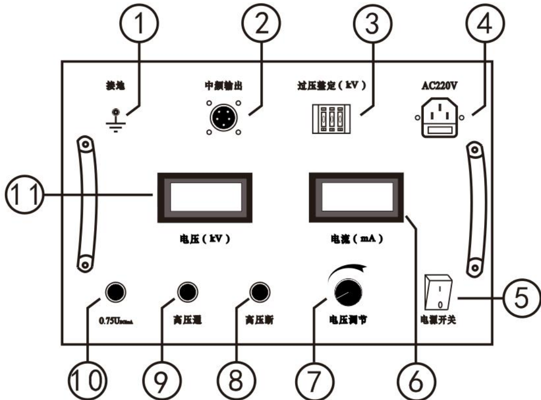
图 2 面板布局图
