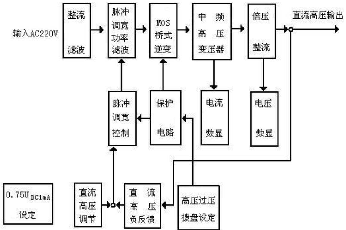
图 1 工作原理图
